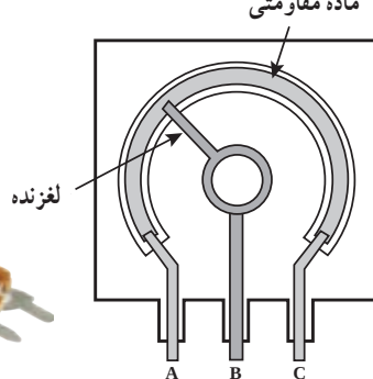
ت) طرحی از یک پتانسیومتر
