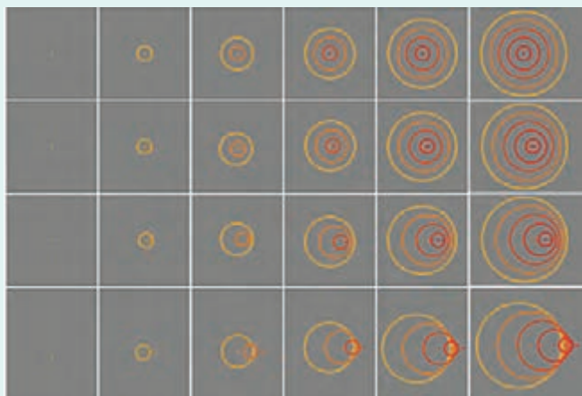
شکل ۲۷-۳ الف) وقتی ماشین ساکن است تجمع جبهه‌های موج در جلو و عقب ماشین یکسان است. ب) با حرکت رو به جلوی ماشین، تجمع جبهه‌های موج در جلوی ماشین بیشتر و در عقب آن کمتر می‌شود.
