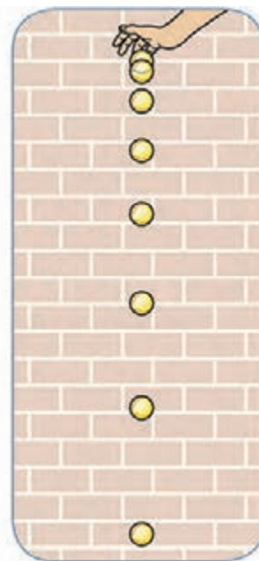
شکل ۱-۱۶ تصویری از یک توپ در حال سقوط آزاد، که در بازه‌های زمانی مساوی و متوالی رسم شده است.
