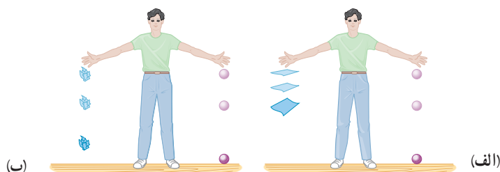
شکل ۱-۱۵ تجربه‌ای ساده برای مقایسه اثر مقاومت هوا روی حرکت سقوط گلوله، برگه کاغذ و برگه کاغذ مجاله شده
