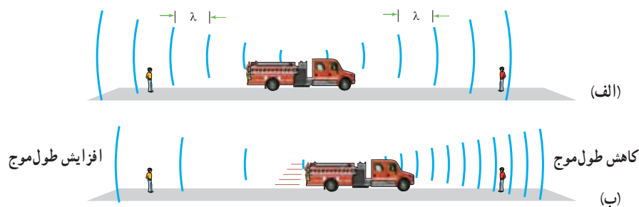
شکل ۲۷-۳ الف) وقتی ماشین ساکن است تجمع جبهه‌های موج در جلو و عقب ماشین یکسان است. ب) با حرکت رو به جلوی ماشین، تجمع جبهه‌های موج در جلوی ماشین بیشتر و در عقب آن کمتر می‌شود.
