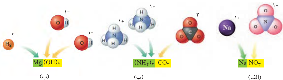
شکل ۶- نام و فرمول شیمیایی (الف) سدیم نیترات، (ب) آمونیوم کربنات و (پ) منیزیم هیدروکسید
