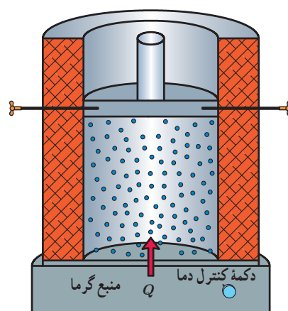
شکل ۵-۷ دمای گاز را در فرایند هم‌حجم با استفاده از منبع گرمایی با دمای قابل تنظیم، به تدریج تغییر می‌دهیم.
