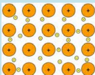
پیوند فلزی
