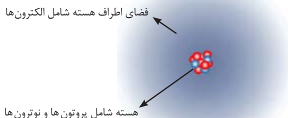
شکل ۱. اتم از هسته و فضای اطراف هسته تشکیل شده است.
