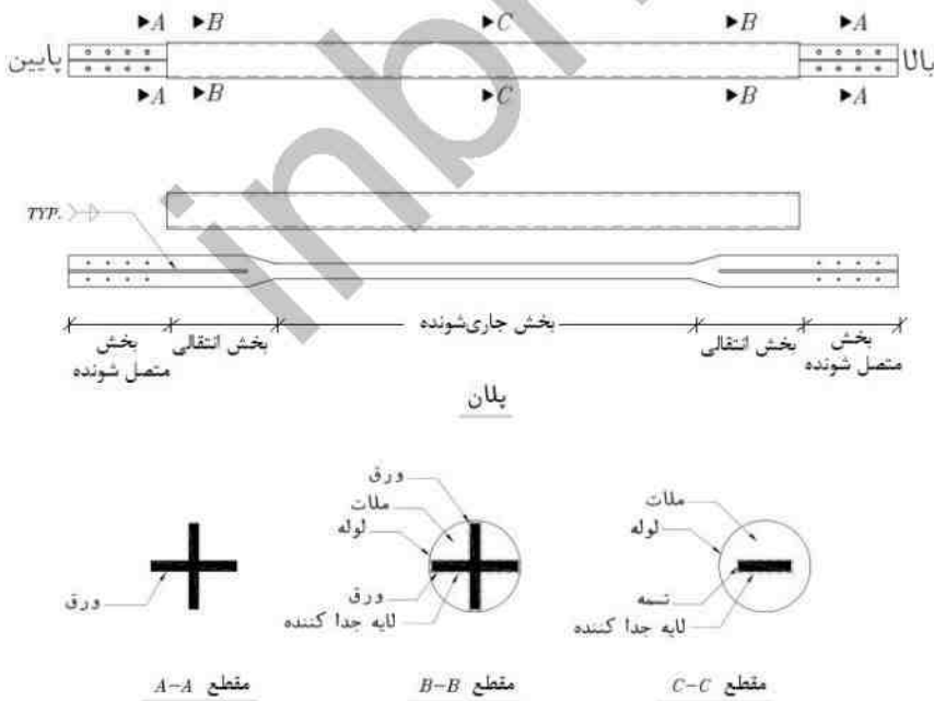
شکل ۳-۱۰-۴-۴: نمونه‌ای از اجزای یک مهاربند کمانش تاب
