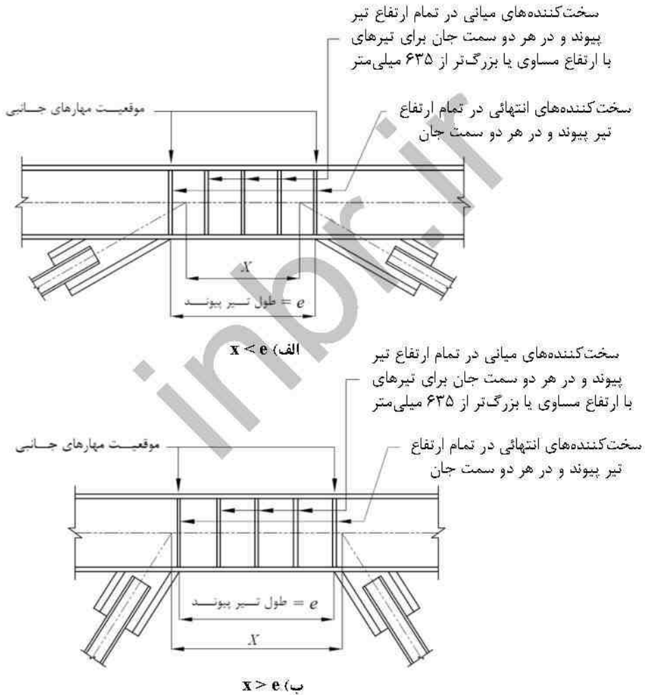
شکل ۱۰-۳-۳-۴-۲: تیر پیوند با مقطع I شکل و سخت‌کننده‌های موردنیاز
