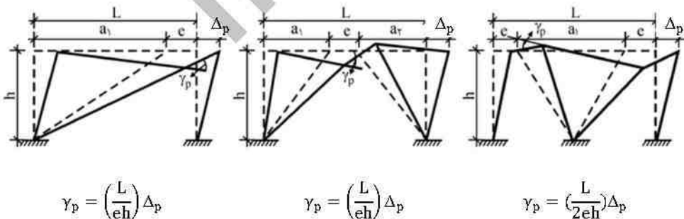
شکل ۱۰-۳-۴-۳-۴: دوران پلاستیک تیر پیوند نسبت به ناحیه خارج از آن ( \gamma_p )
