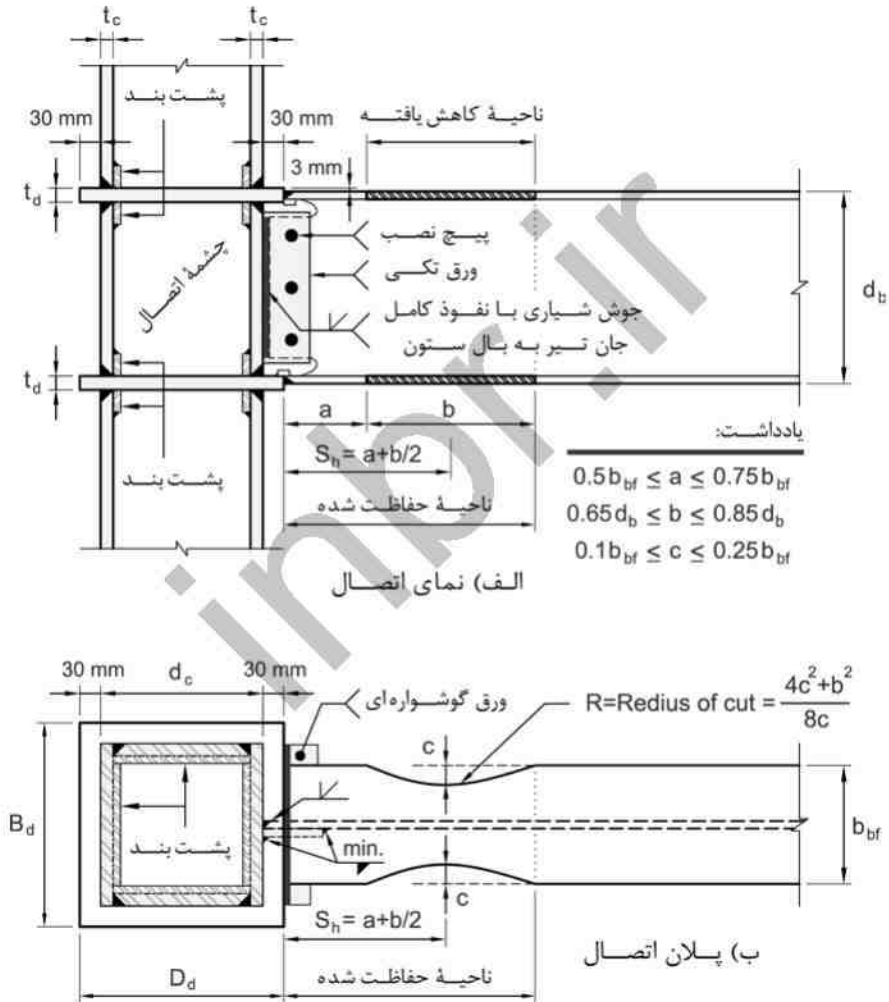
شکل ۱۰-۳-۷-۱۰: اتصال گیردار تیر با مقطع کاهش یافته و دیافراگم عبوری از ستون (TD-RBS)
