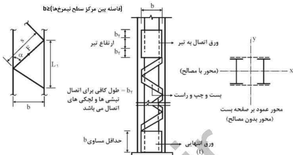
شکل ۲-۱۰-۳-۴-۳: عضو فشاری ساخته شده (مکعب) با بست‌های مورب
