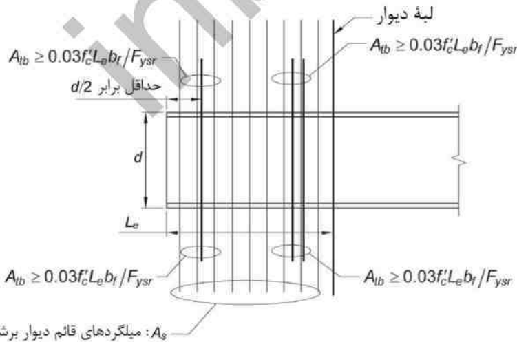
شکل ۳-۶-۳-۱۰-۲: میلگردهای قائم دیوار و میلگردهای انتقال در محدوده طول مدفون تیر همبند
