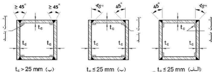
شکل ۱۰-۳-۷: نحوه ساخت ستون‌های جعبه‌ای ساخته شده از ورق
