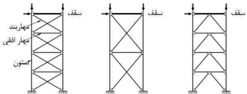
مهاربند چند ردیفی ضربدری مهاربند دو ردیفی ضربدری مهاربند چند ردیفی از نوع A
