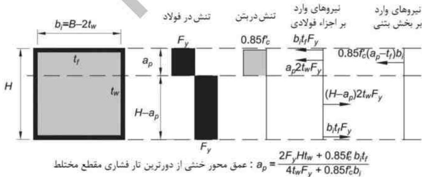
شکل ۱۵-۸-۲-۱۰: محاسبه لنگر خمشی پلاستیک مقطع مختلط پر شده با بتن برای مقاطع فشرده
