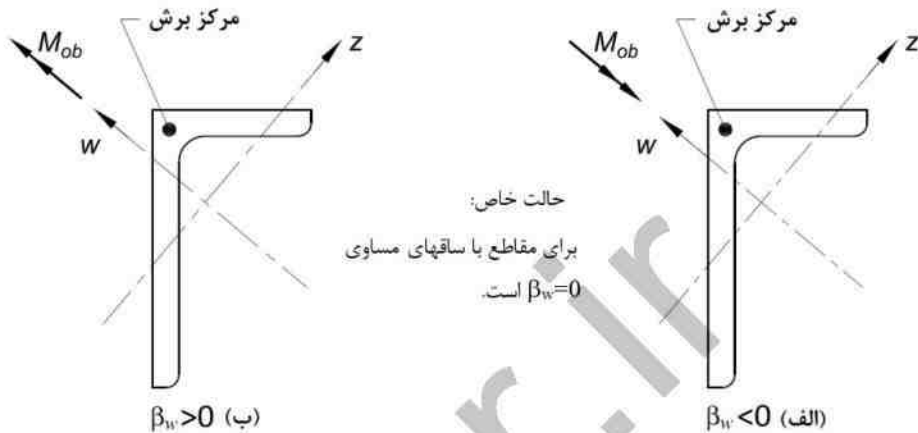
شکل ۱۰-۲-۵-۱: مشخصات مقطع نبشی تک و علامت مثبت یا منفی \beta_w
