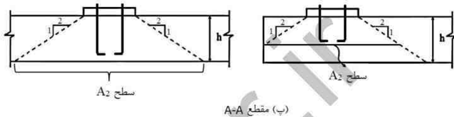
شکل ۲-۱۰-۳-۹-۲۲: سطح اتکا در تماس با تکیه‌گاه بتنی
