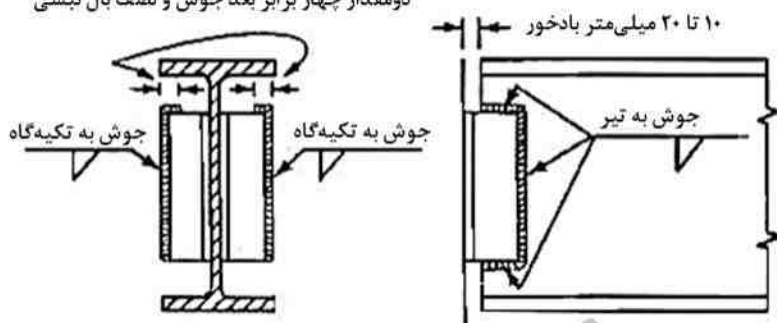
شکل ۱۰-۳-۵: جزئیات اتصال جوشی با استفاده از نبشی جفت در جان
