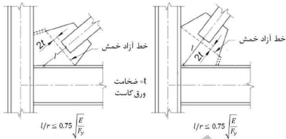
شکل ۳-۱۰-۲-۴-۳: سازگاری ورق اتصال (ورق گاست) با کمانش خارج از صفحه عضو مهاربندی
