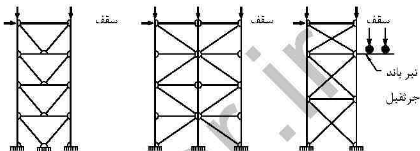
مهاربند چند ردیفی از نوع V مهاربند چند ردیفی دو دهانه مهاربند چند ردیفی ضربدری
