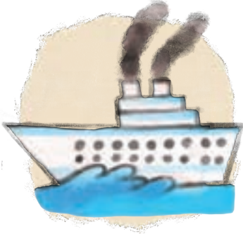
کشتی
