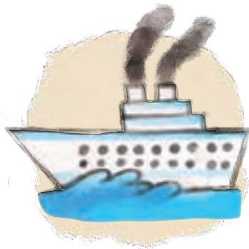
کشتی
