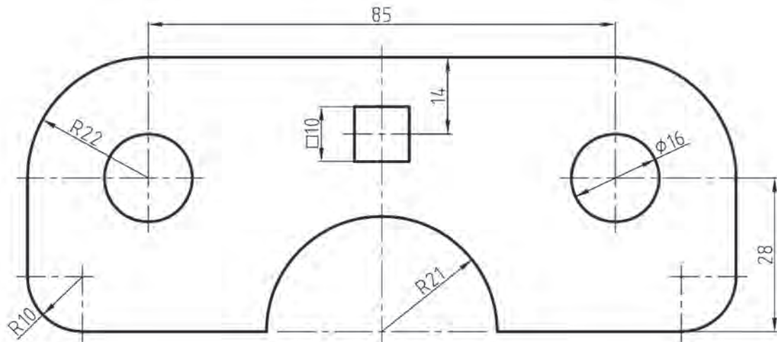
شکل ۸-۲۸. اندازه گذاری نقشه
