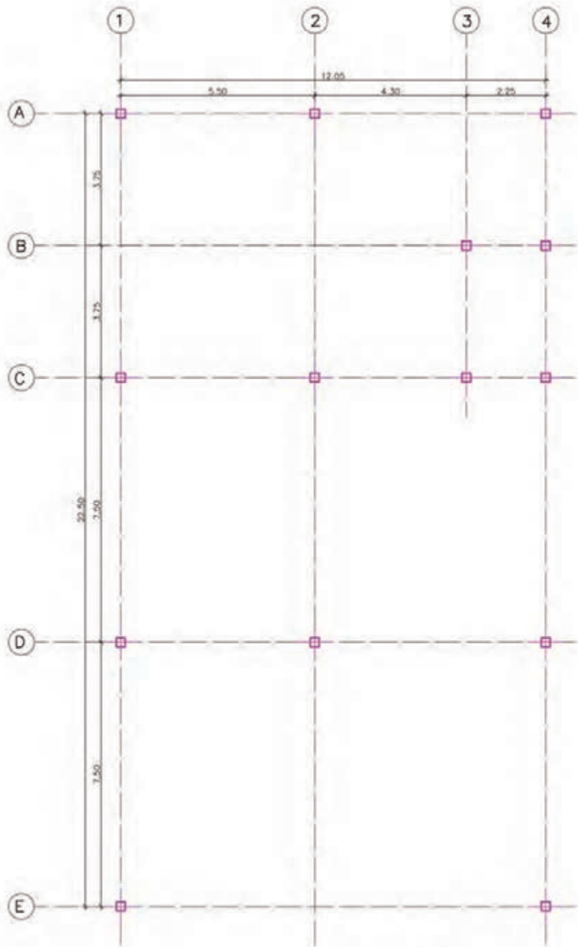
مرحله ۳-۲ قرارگیری ستون ها روی محورها
