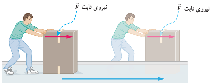
شکل ۳-۱ نیروی ثابت \vec{F} که با جابه جایی \vec{d} هم جهت است، کار W = Fd را انجام می دهد.
