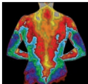
شکل ۴-۳۳ تصویری دمانگاشت از بدن یک فرد. سطح بدن یک فرد معمولی با دمای 37^{\circ}\text{C} ، در محیطی با دمای 20^{\circ}\text{C} به دلیل تابش گرمایی، با آهنگی در حدود 70\text{W} گرما از دست می‌دهد.
