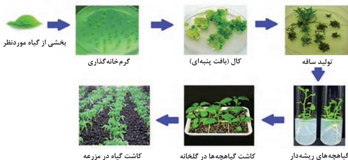
شکل ۲۵- مراحل کشت بافت. از یک برگ کوچک با کشت بافت می توان تعداد زیادی کال (بافت پنبه ای) به دست آورد. این کال ها به گیاهچه های دارای ساقه و ریشه تبدیل می شوند.
