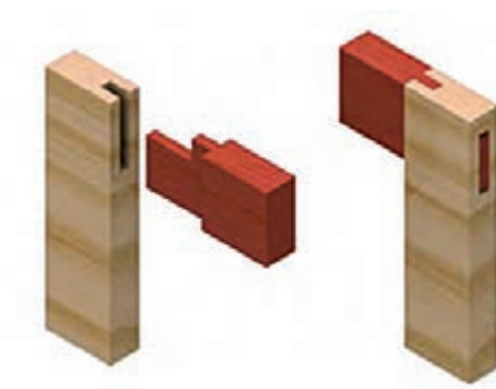
شکل ۲۵- اتصال کام و زبانه
