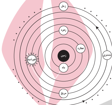
شکل ۱-۲- نمایش نظریه زمین مرکزی
