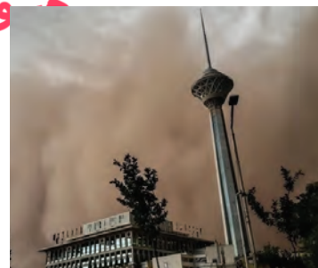
شکل ۱۰-۵. توفان گرد و غبار
