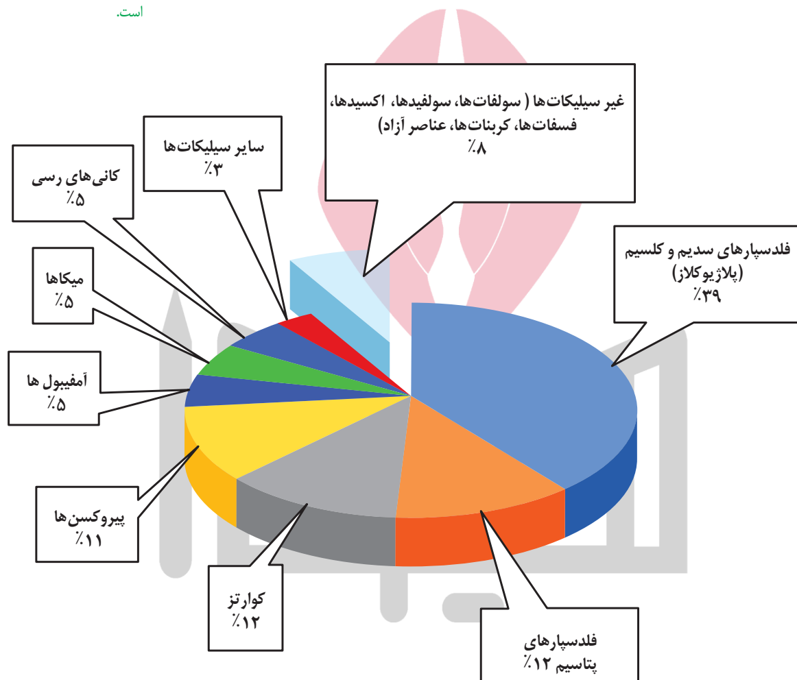
شکل ۲-۲. درصد وزنی کانی‌های سازنده پوسته زمین
