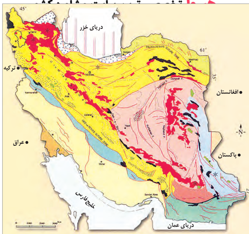
شکل ۷-۲. نقشه پهنه بندی زمین شناسی در ایران
