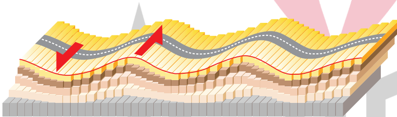
شکل ۴-۶- نحوه حرکت موج سطحی L
