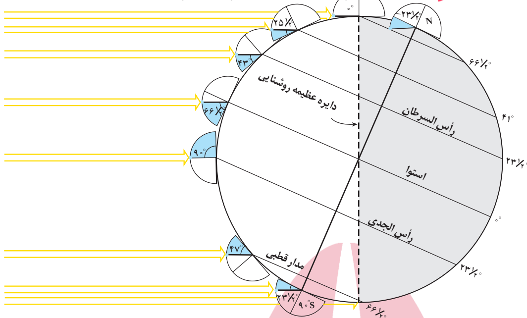
شکل ۴-۱. مقدار انحراف محور زمین و تأثیر آن در مقدار زاویه تابش خورشید در عرض های جغرافیایی مختلف
