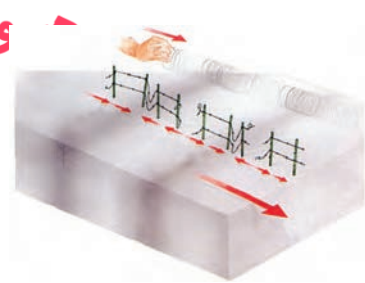
(الف) امواج طولی (P)
