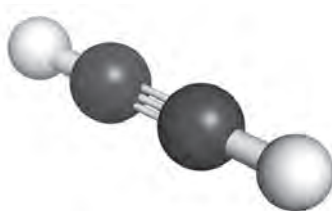
شکل ۶. ساختار فضایی استیلن
