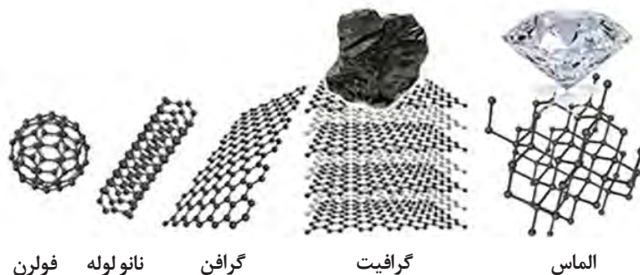
شکل ۱. آلوتروپ‌های کربن
