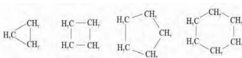
سیکلوپروپان سیکلوبوتان سیکلوپنتان سیکلوهگزان
