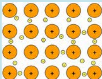
پیوند فلزی
