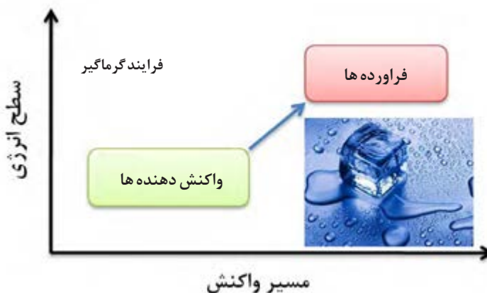
شکل ۸. سطح انرژی واکنش دهنده‌ها و فراورده‌ها در یک فرایند گرماگیر
