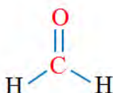
شکل ۱۳. ساختار فرمالدهید. از آن، برای نگهداری موجودات و ساختارهای زنده استفاده می‌کنند.
