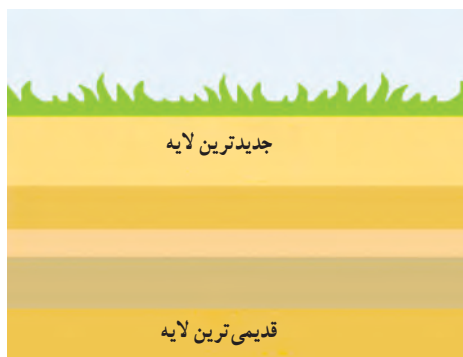
شکل ۱۳- نحوه تشکیل توالی از لایه‌های رسوبی
