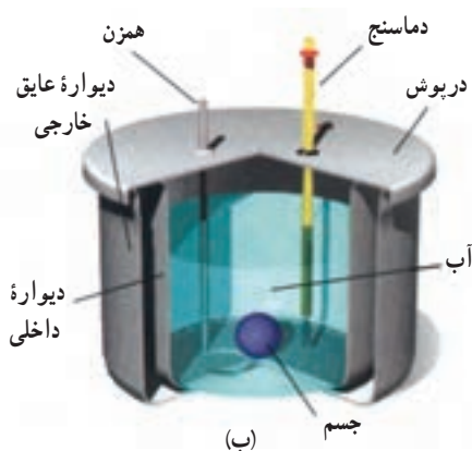
شکل ۱۴-۱۹ (الف) عکسی واقعی و (ب) طرحی از نمای داخلی یک گرماسنج
