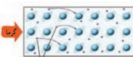
الکترون‌های آزاد
