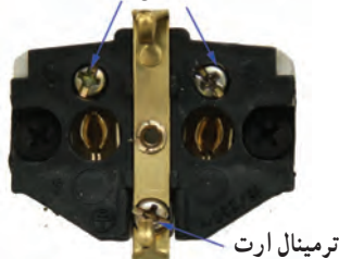
شکل ۵-۱۲- استفاده از اتصال ارت
