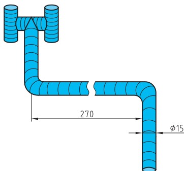
خ - استفاده از دودکش با قطر کمتر از ۱۵ سانتی متر برای آبگرمکن دیواری یا پکیج شوفاز دیواری مجاز نیست.
