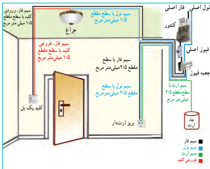
شکل ۵-۶ - سیم کشی مدار یک پل
